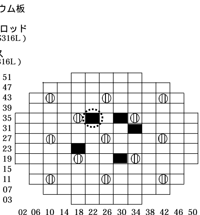
ハフニウム板型制御棒の炉内での位置
