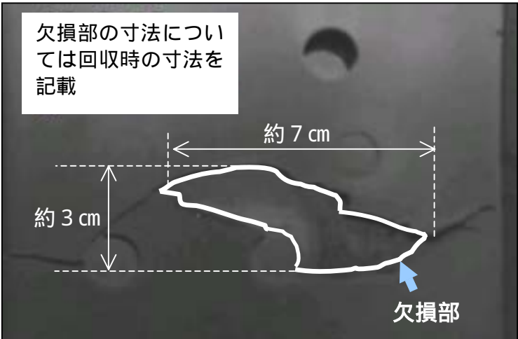
制御棒のシース部で確認されたひびおよび欠損部の状況
