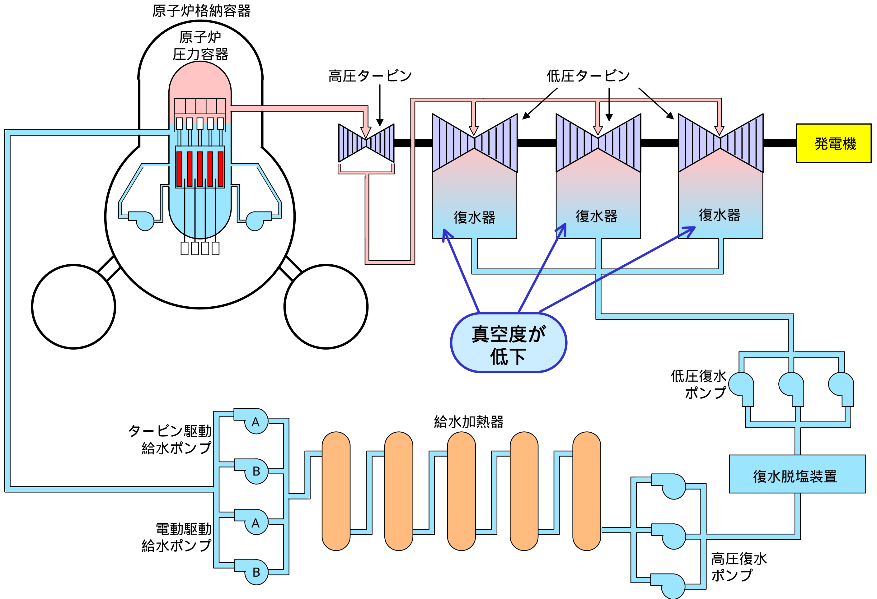
4号機系統概要図
