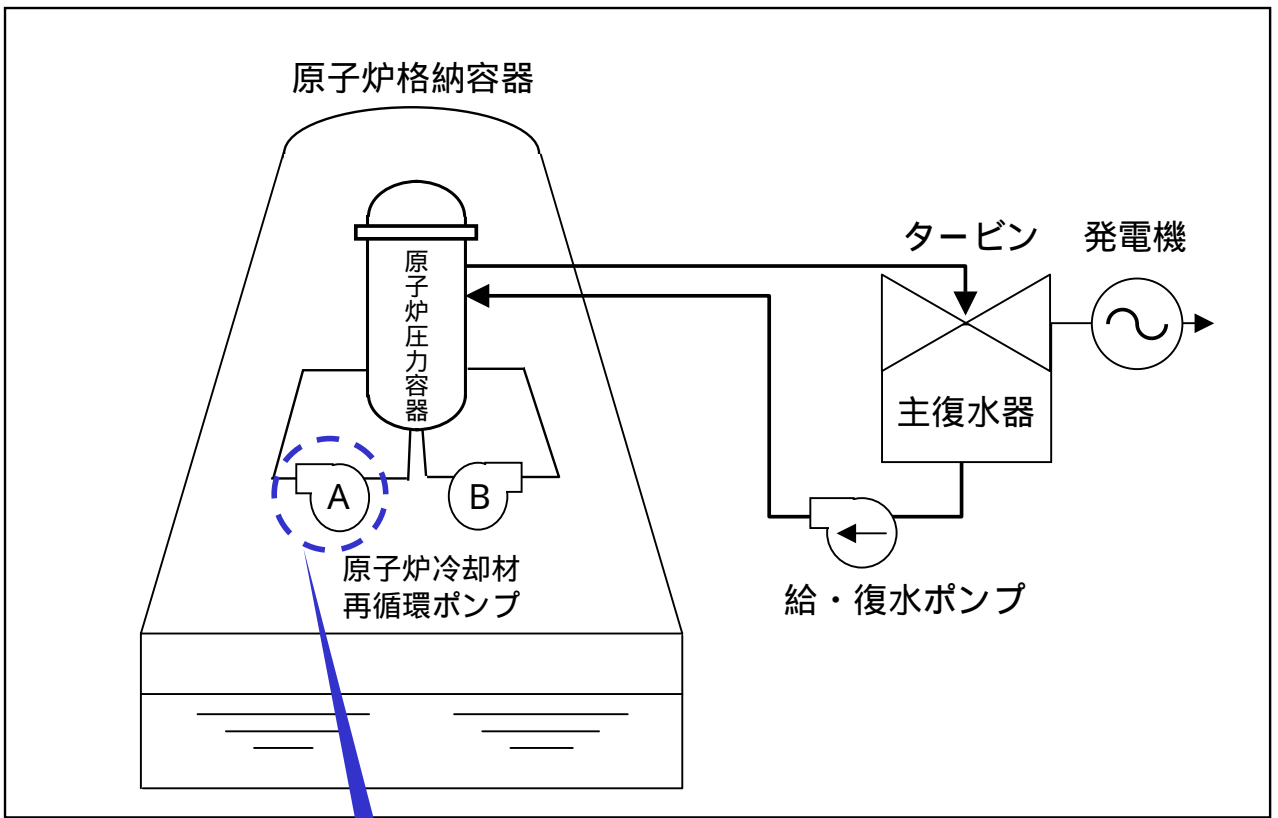
系統概略図
