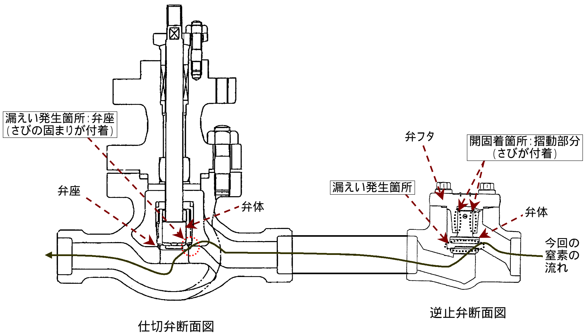
事象発生時の当該弁の状態および窒素の流れ図
