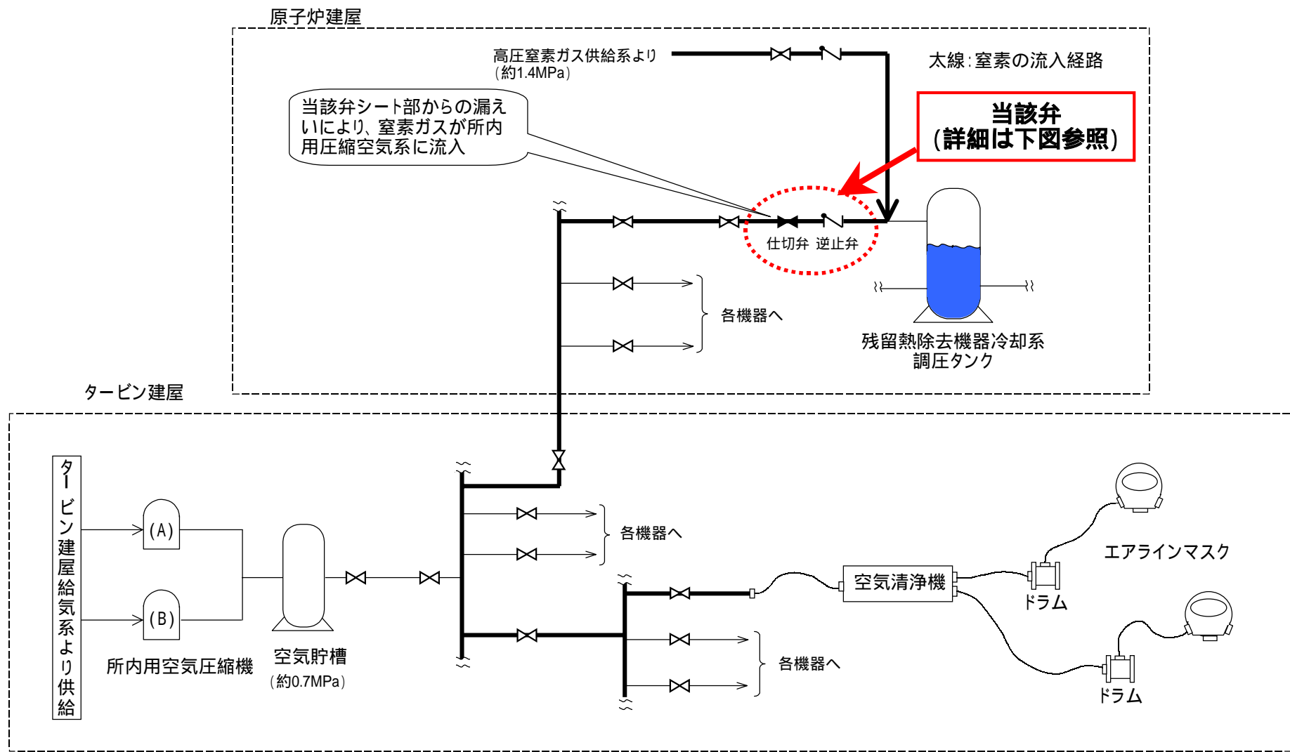
福島第二原子力発電所4号機 所内用圧縮空気系 概略図
