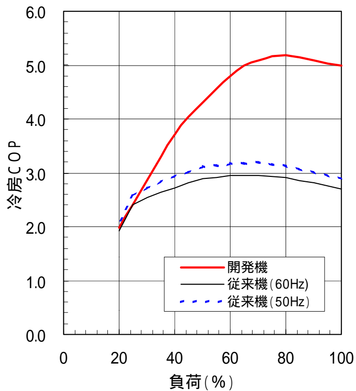
図2. 部分負荷特性
