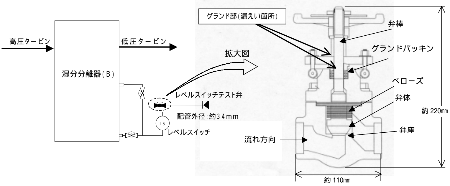
1 湿分分離器概略図及びレベルスイッチテスト弁構造図
