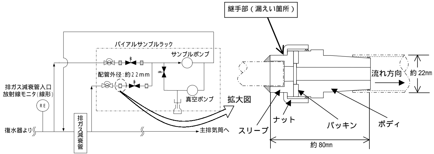
2 排ガス減衰管バイアルサンプルラック概略図及び継手部構造図
