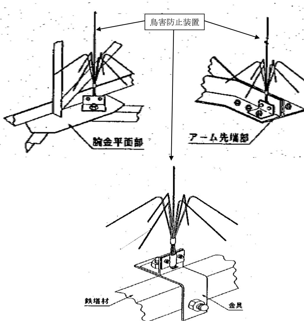
【鳥害防止装置①】
