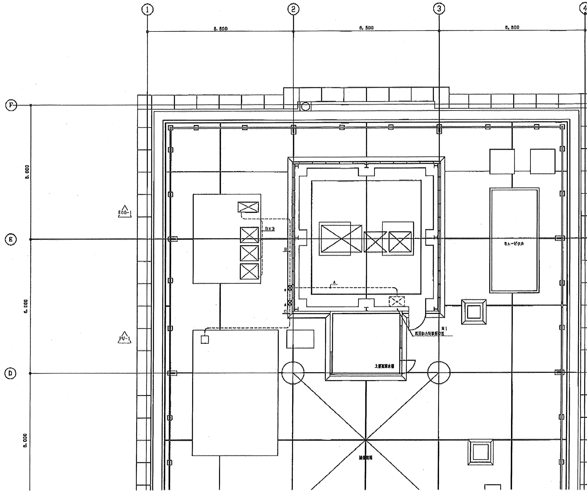
R階平面図 S=1/50
