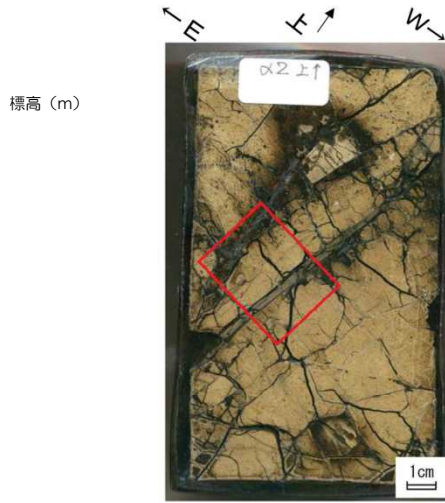
薄片試料採取位置
