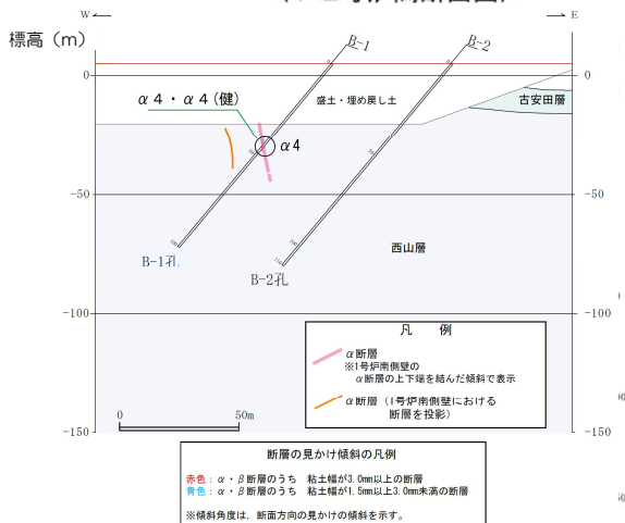
X線回折分析試料採取位置図 (1号炉南方面断面図)
