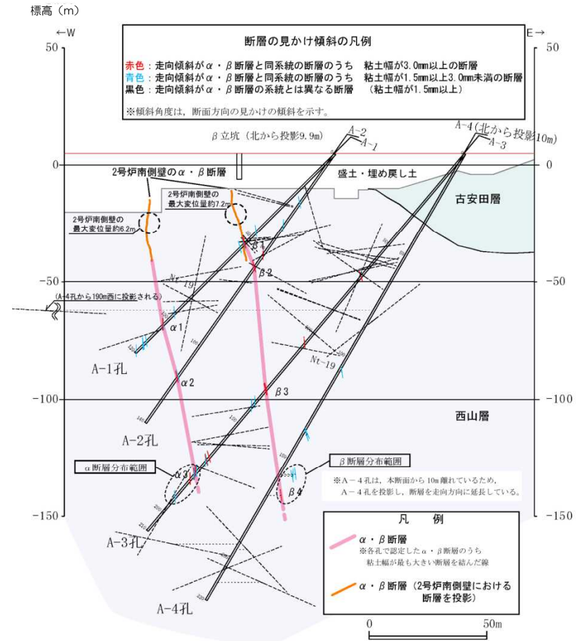
断層の連続性
