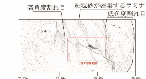
F5-11孔 掘削深度25.85～26.00mスケッチ
