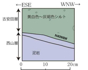
境界2 試料採取面スケッチ
