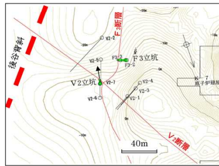
V2立坑付近の西山層上限面の全体的な傾斜方向 V2立坑位置図
