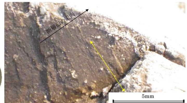
\beta 断層 ( \beta 2 )の条線 (黄色矢印方向) 断層面の走向・傾斜: N4E75E 条線のレイク角: 90
