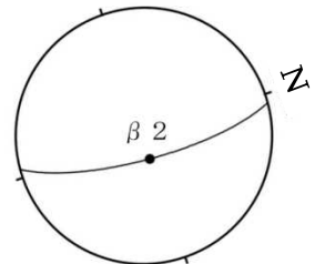
\beta 2 の走向・傾斜と条線方向 (シュミットネット下半球投影)
