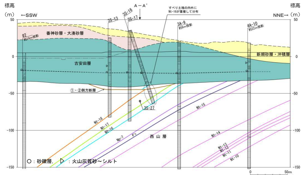
6-6' 断面図
