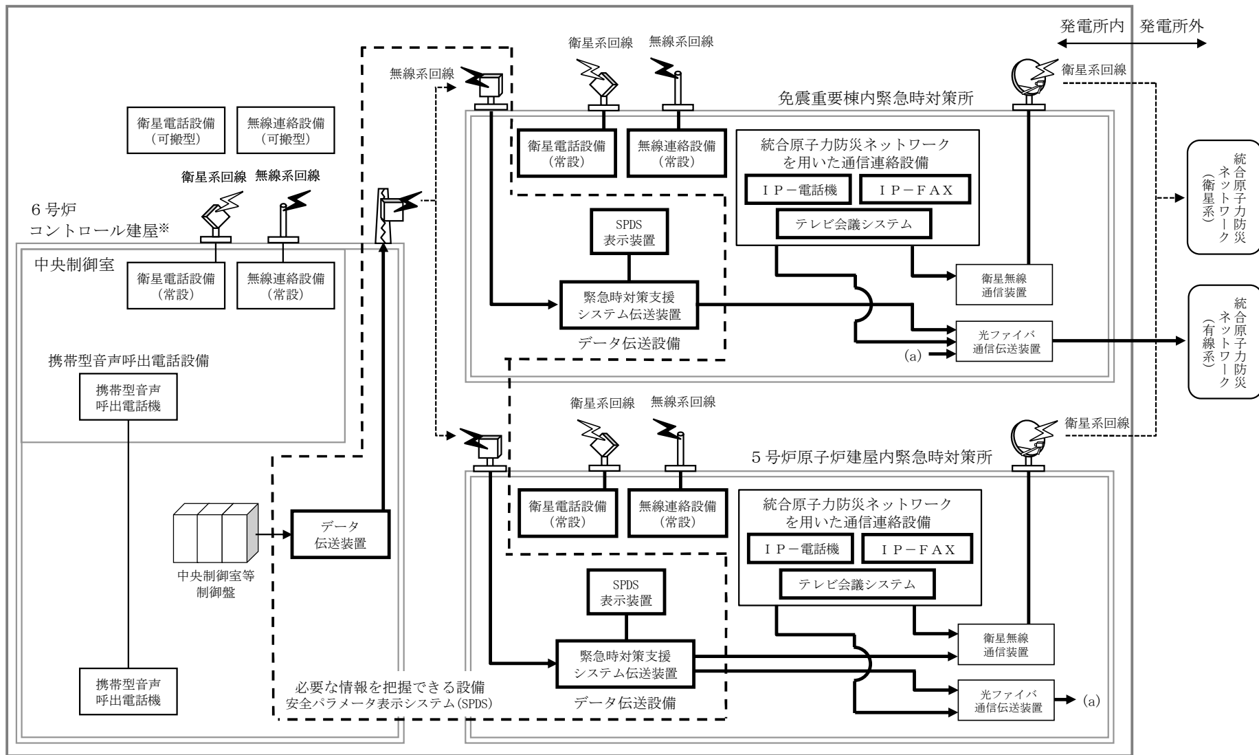
図 3. 18. 2. 4. 1-1 必要な情報を把握できる設備及び通信連絡設備(5号炉原子炉建屋内緊急時対策所) 概略系統図
