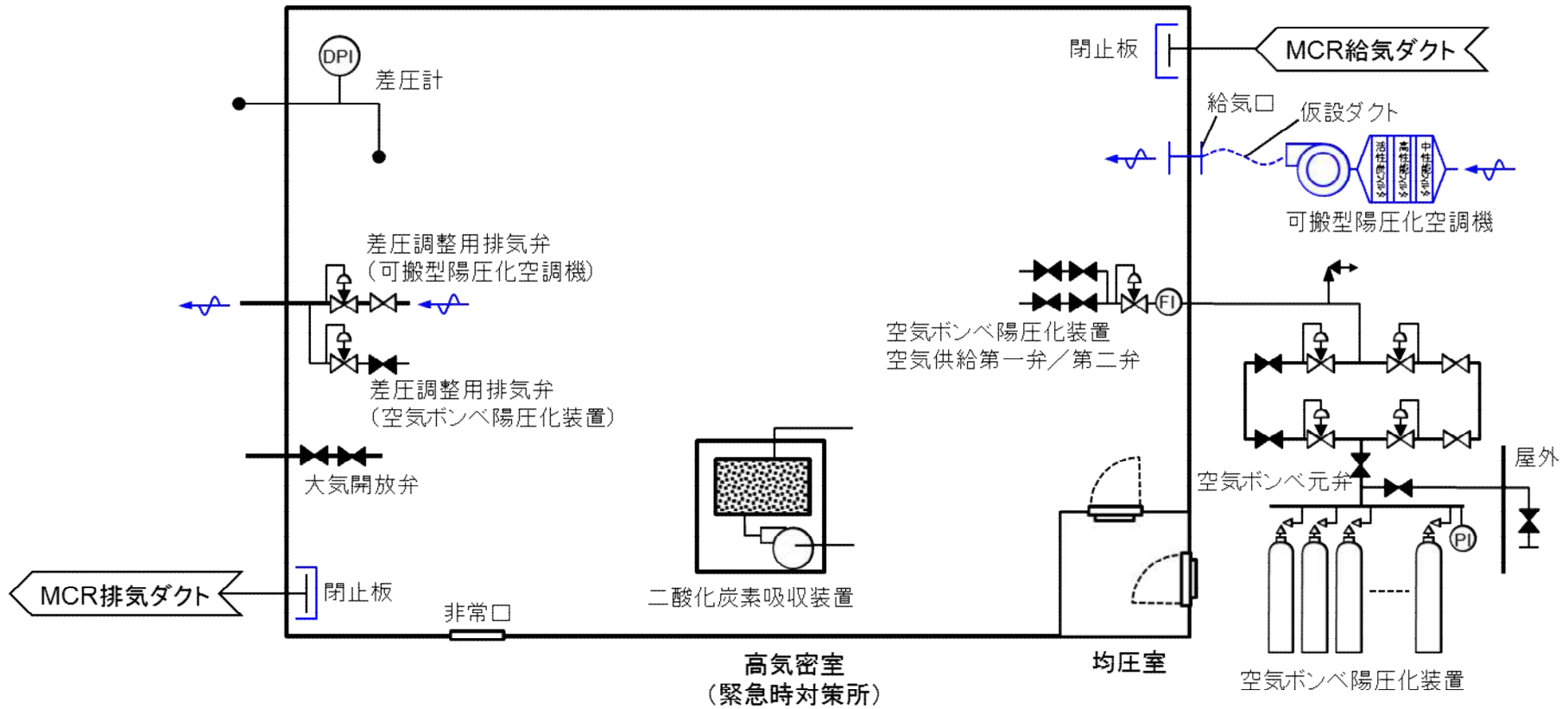
図 3. 18. 2. 6. 1-1 5号炉原子炉建屋内緊急時対策所換気設備 系統概略図 (プルーム通過前後：可搬型陽圧化空調機による陽圧化時)
