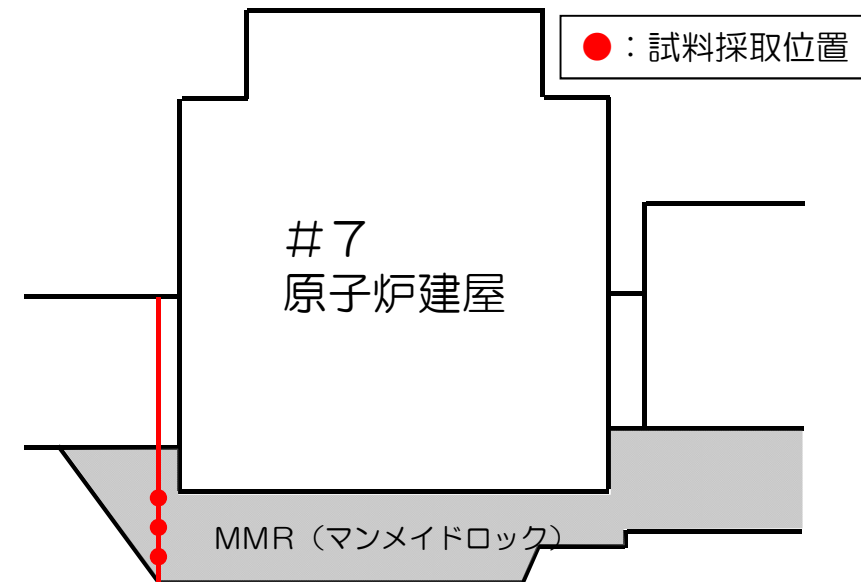
A-A'断面図
