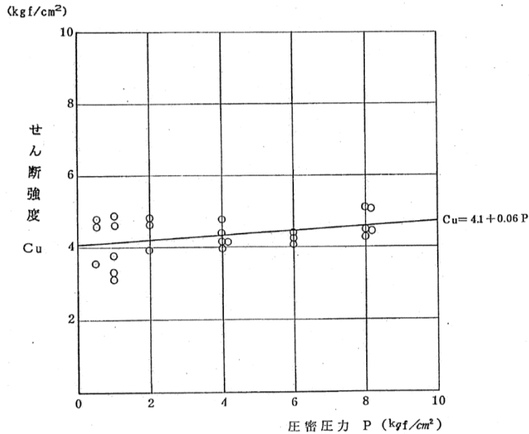
F_5 断層（粘土部）のせん断強度
