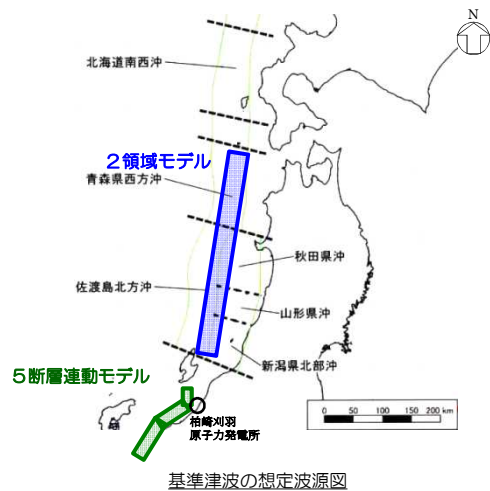
基準津波の想定波源図
