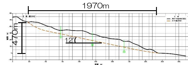
断面図
