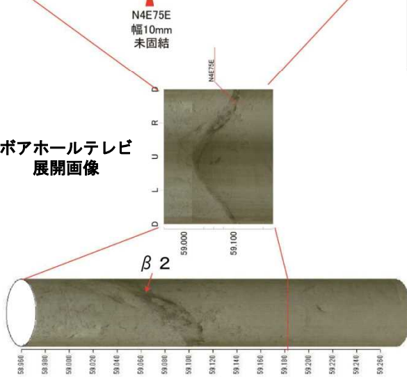
ボアホールテレビ孔壁画像
