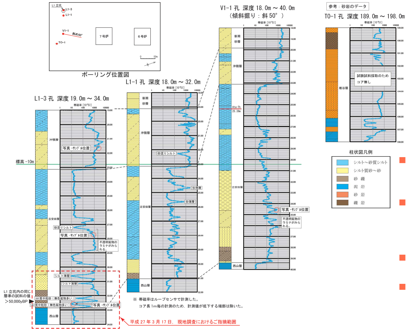
帯磁率測定結果
