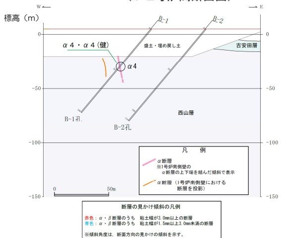
X線回折分析試料採取位置図 (1号炉南方断面図)
