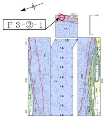
F3-②-1 試料採取位置
