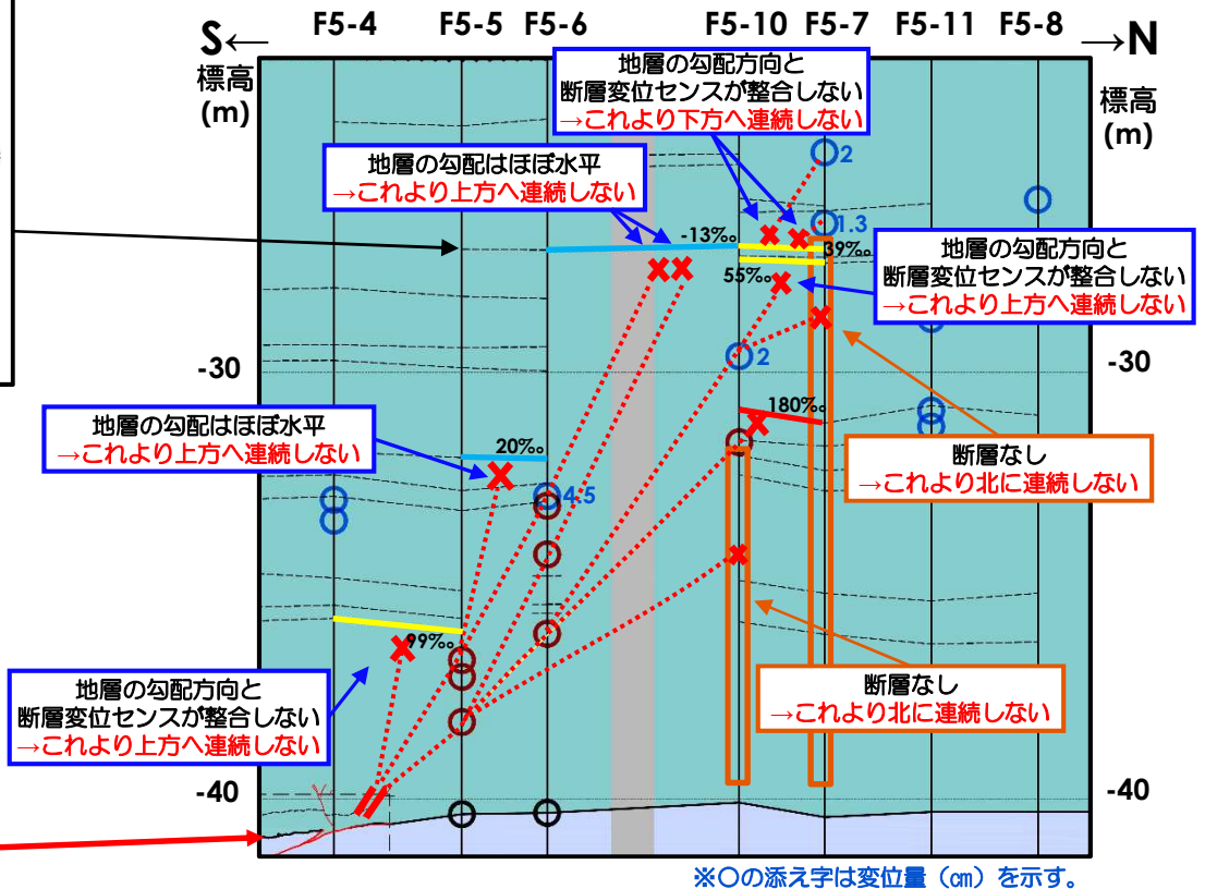
F5立坑近傍の地質断面図 (拡大)
