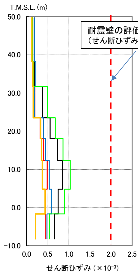
建屋のせん断ひずみの比較 (Ss-1, NS方向)
