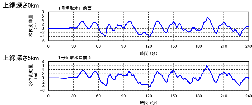
1号炉取水口前面水位変動量 時刻歴波形
