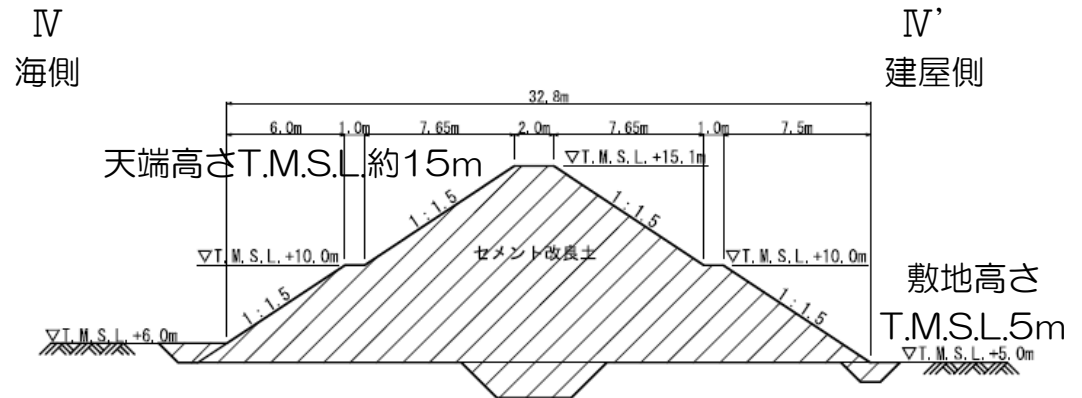
セメント改良土 (Ⅳ-Ⅳ' 断面)
