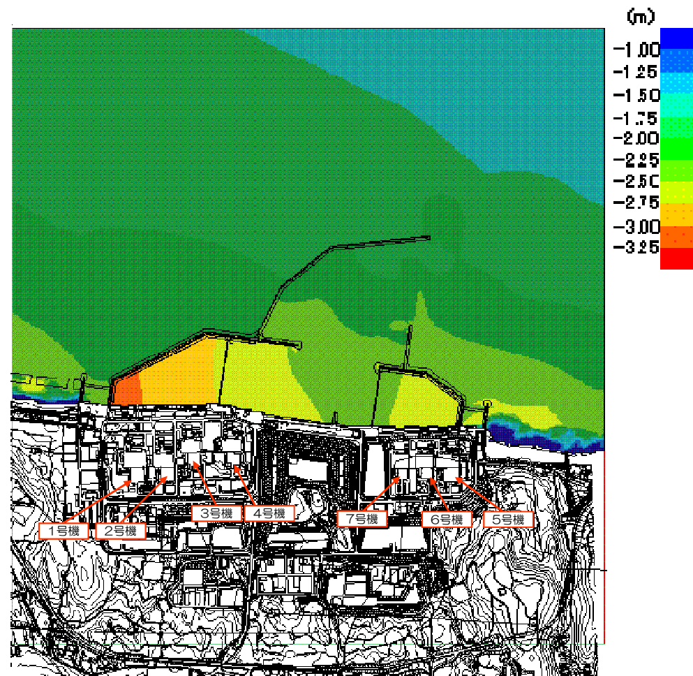
最大水位下降量分布図
