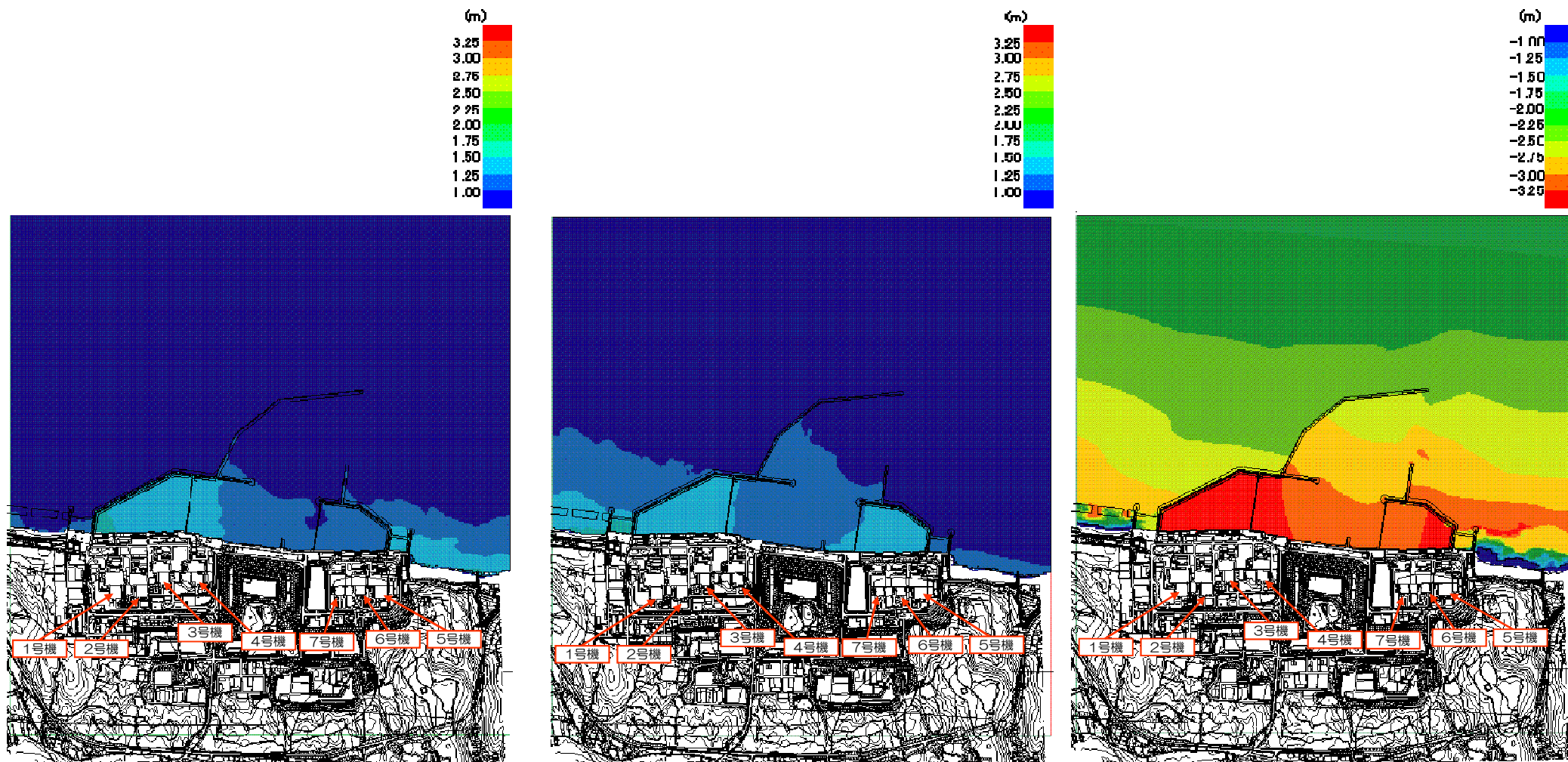
最大水位上昇量分布図（1～4号機）
