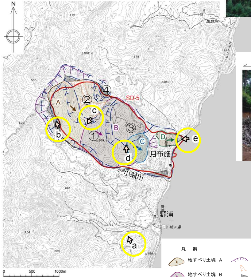
地すべり全景写真 a 比較的緩やかな地すべり土塊。 小瀬川が地すべり土塊を規制する。
