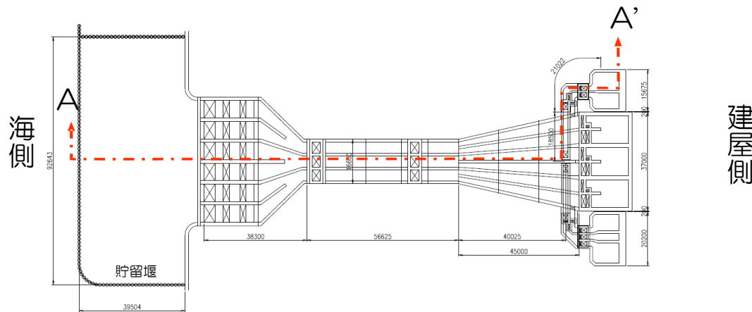
6号炉取水路平面図
