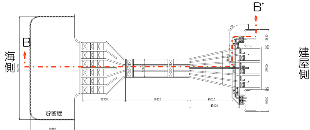
7号炉取水路平面図
