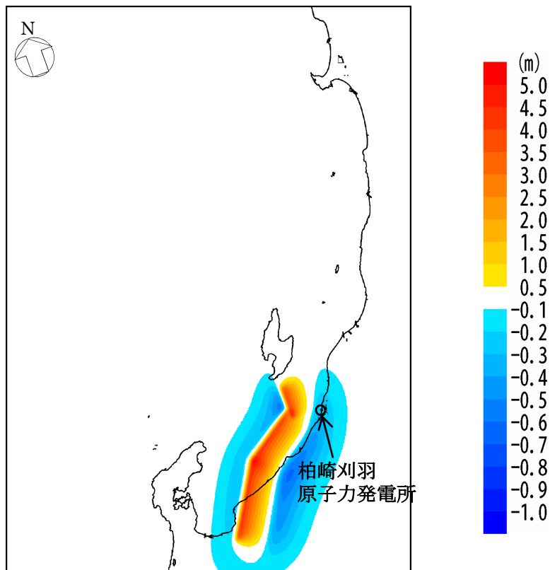
遡上域最大水位ケース： 海域の活断層（5断層連動モデル）＋地すべり（LS-2）
