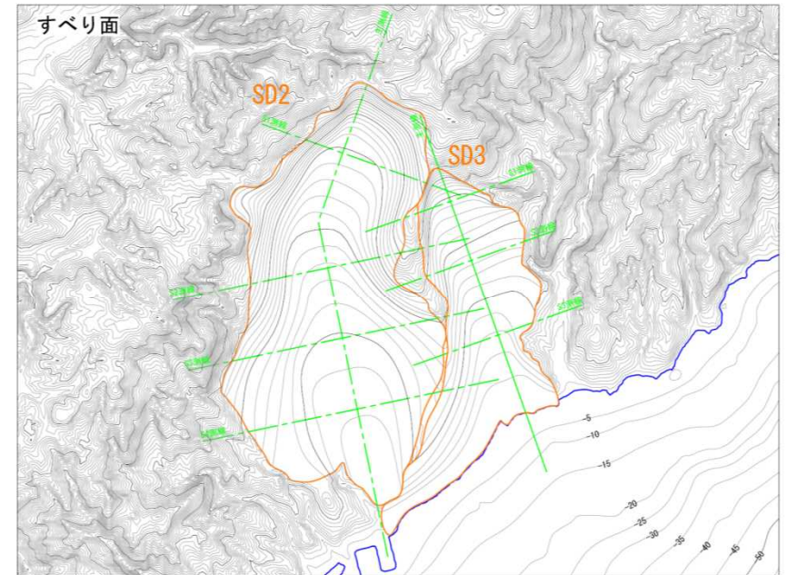
推定したすべり面
