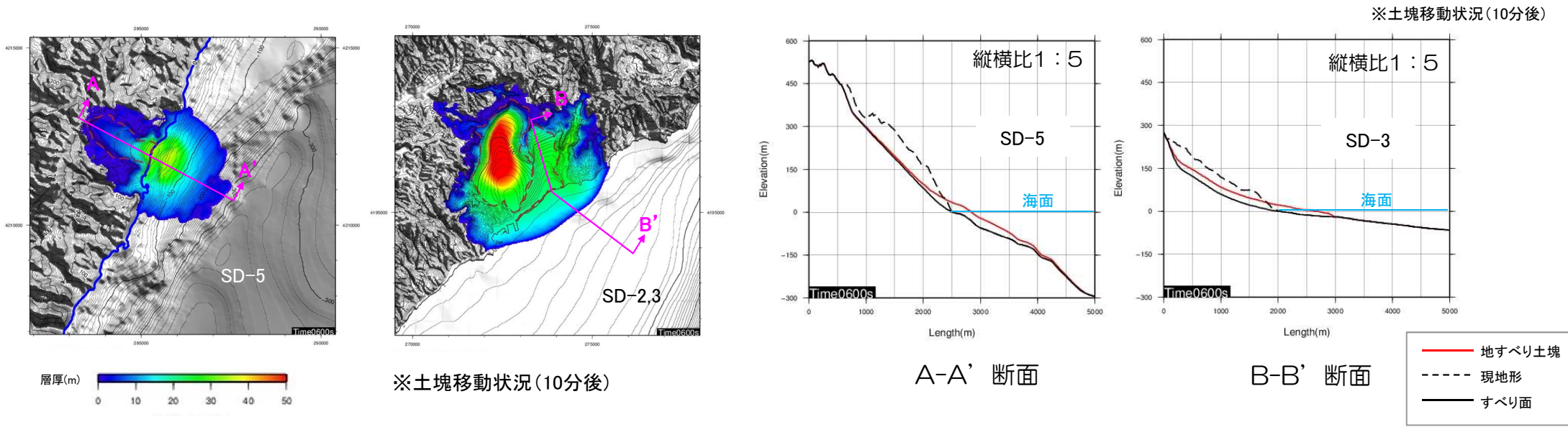
SD-5, SD-2,3の比較 (左：土塊移動状況, 右：海底地形)
