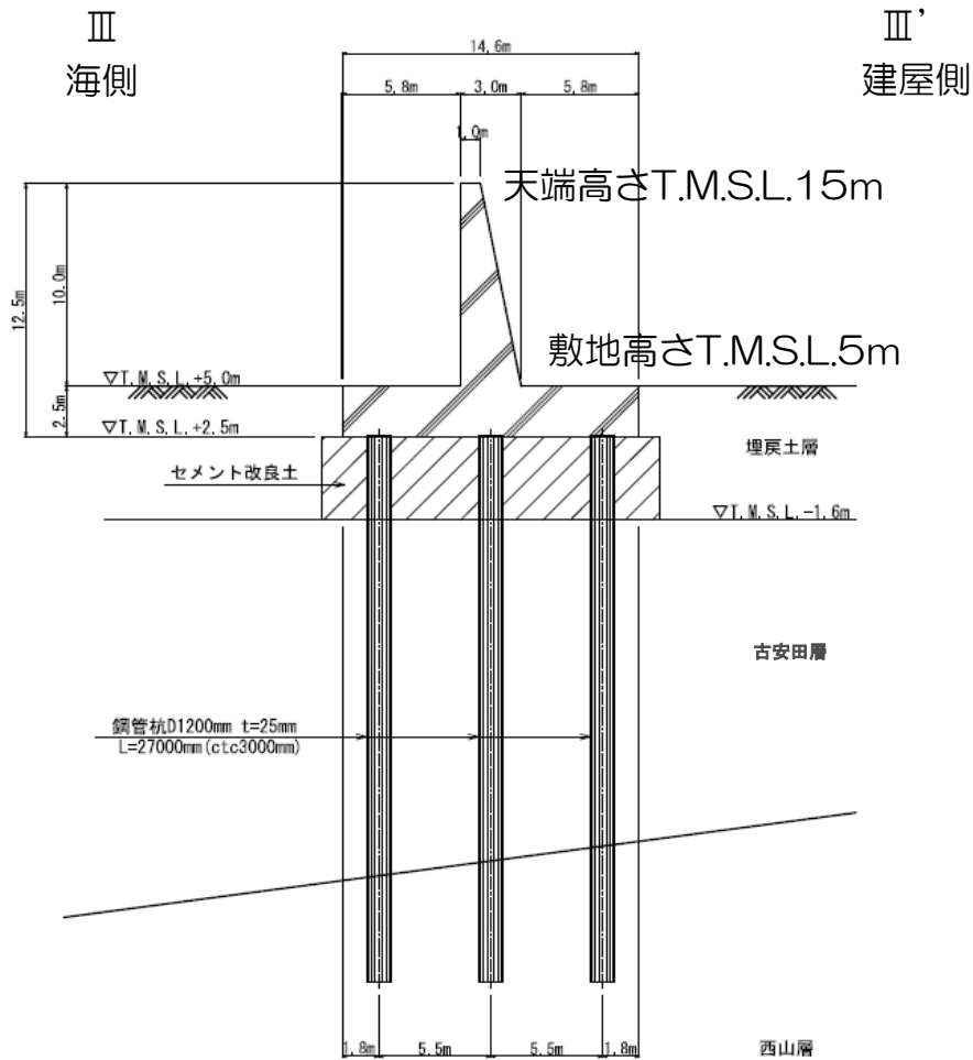
鉄筋コンクリート造 (Ⅲ-Ⅲ' 断面)
