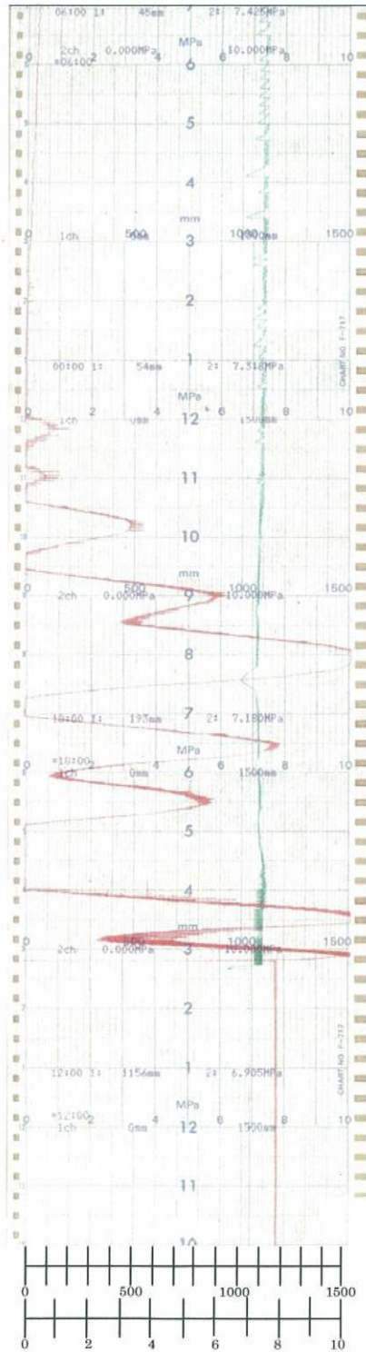
図 12. 福島第一原子力発電所 3号機 原子炉水位と原子炉圧力の変化 *3
