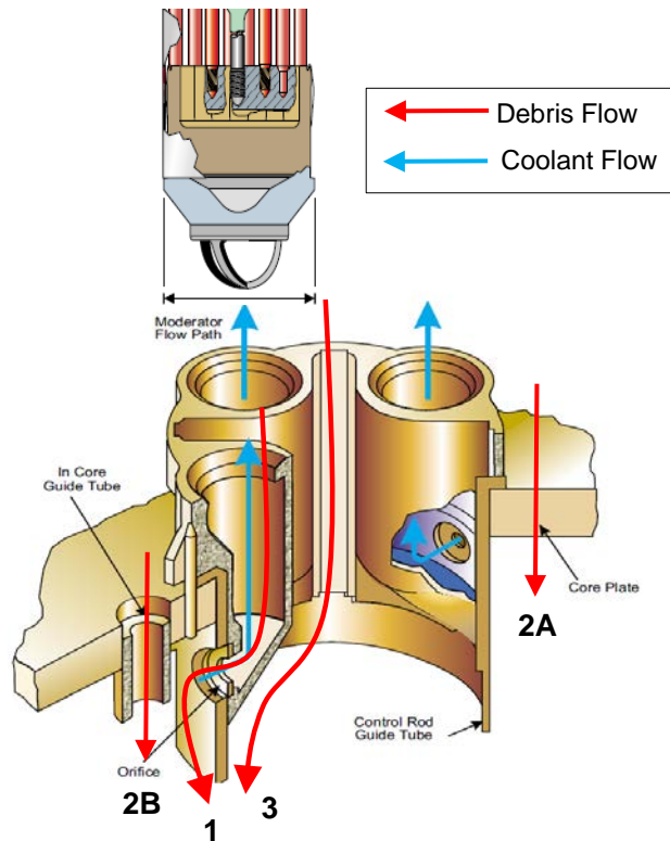
別図 1-2.2-4 炉心下部構造物を介した熔融炉心の移行経路 [4]
