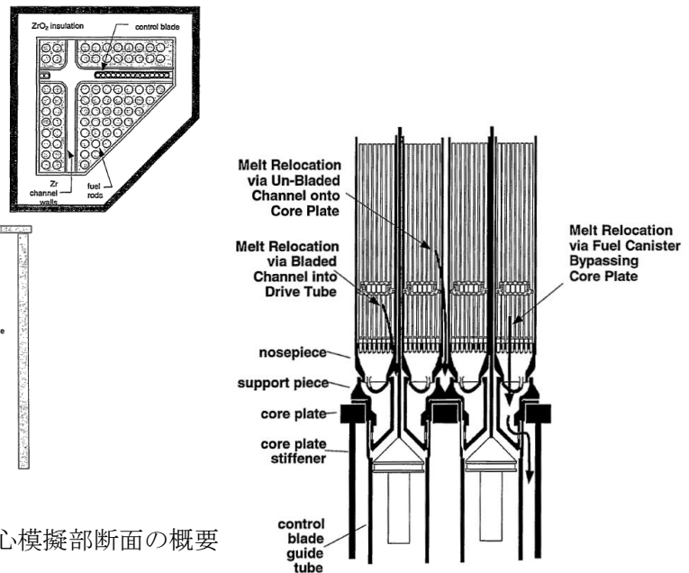
別図 2-2-2 炉心熔融物の流出経路の概要
