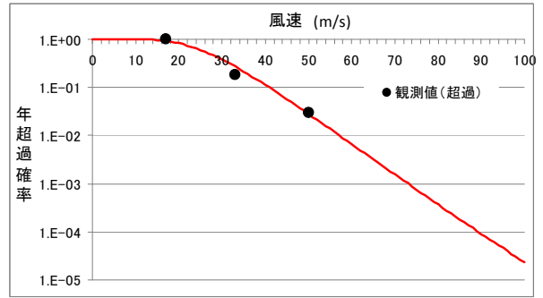
図2.3.5.2 竜巻風速の年超過確率分布
