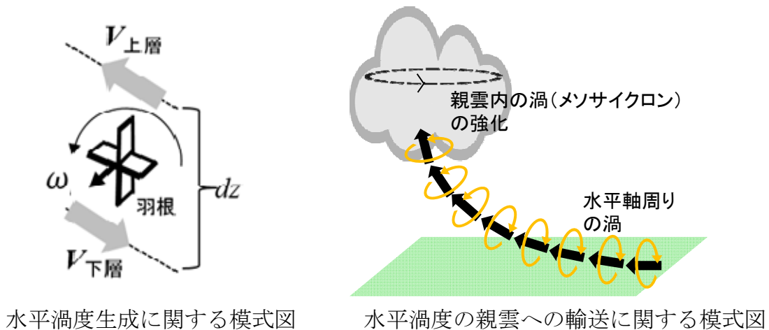
図 2. 2. 4. 3 SReH の算出概念
