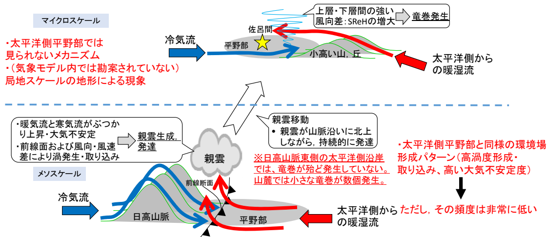
図 2. 2. 4. 13 佐呂間竜巻の発生メカニズムに関する模式図
