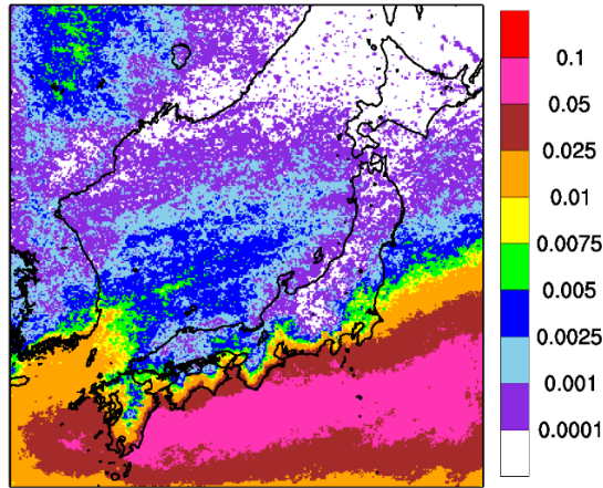
図2. 2. 4. 8 EHIの超過頻度分布（単位：％）
