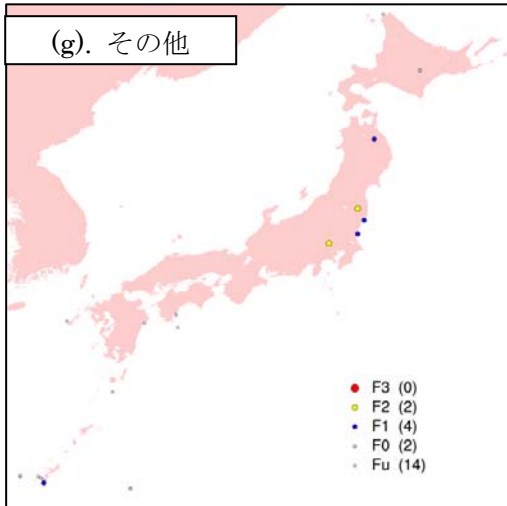
図 2.2.2(続き) 総観場ごとのスケール別竜巻発生地点の分布 (1961年～2012年)
