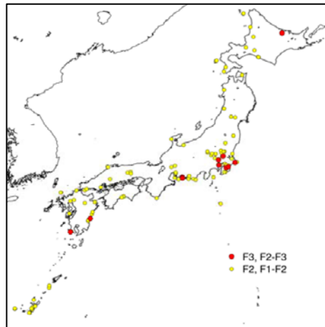
図 2.2.3 F2以上の竜巻発生箇所
