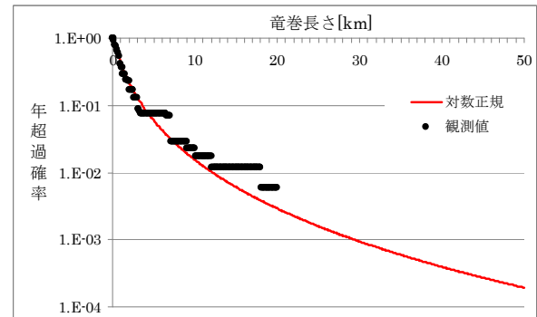
図2.3.5.6 被害長さの年超過確率分布
