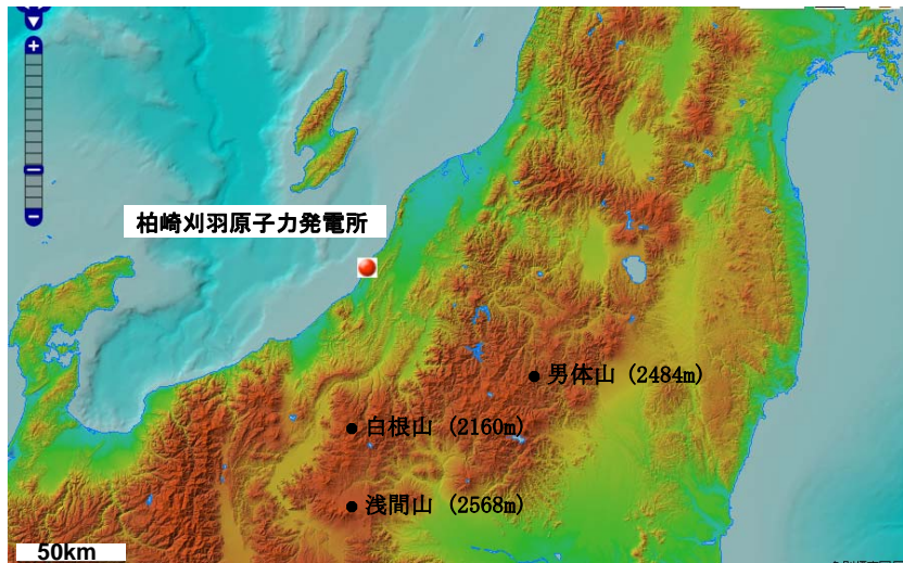
図2. 2. 4. 14 柏崎刈羽原子力発電所周辺地形図
