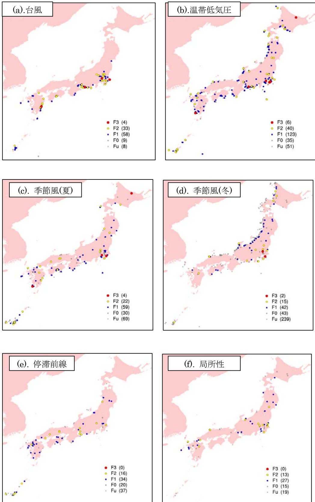
図 2.2.2 総観場ごとの竜巻発生地点の分布(1961年～2012年)
