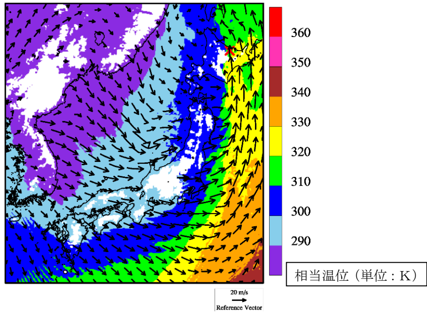
図 2. 2. 4. 11 佐呂間竜巻発生時の風向・風速および相当温位の分布 (海拔 500 m 高度)
