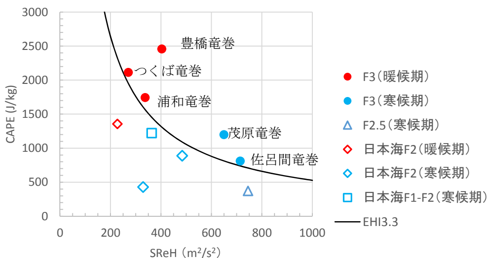
図 2.2.4.5 F3 竜巻, F2-F3 竜巻, および日本海側 F2 竜巻における SReH と CAPE の関係
