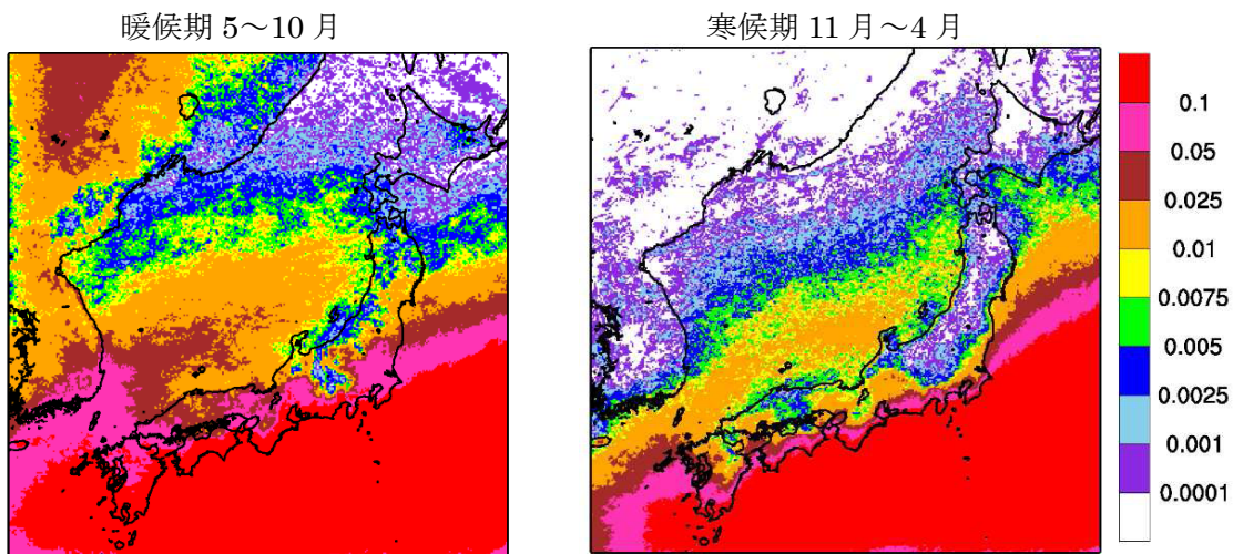
図2. 2. 4. 9 F2規模のSReH，CAPE同時超過頻度分布（単位：％）
