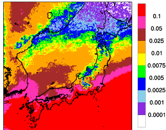
図2. 2. 4. 10 EHIの超過頻度分布（単位：％）
