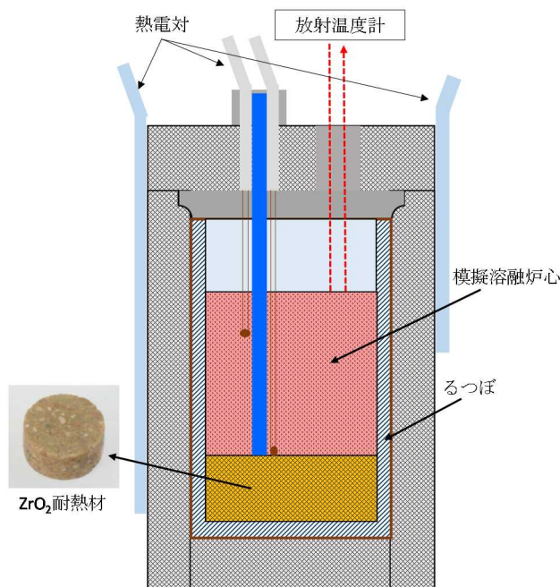
図別 - 3 試験体系
