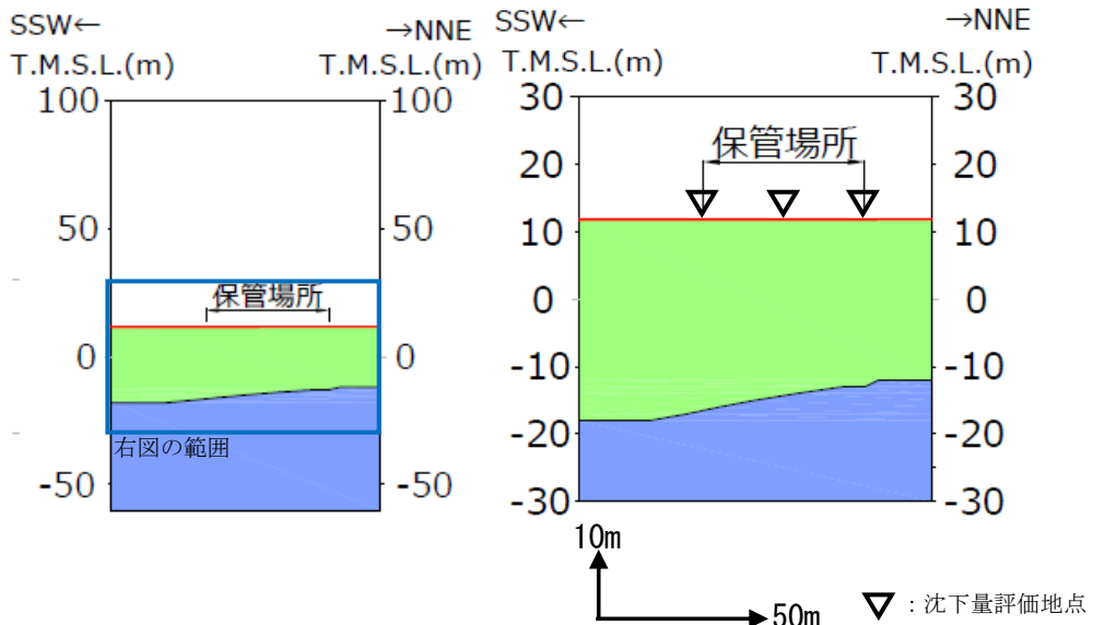
断面位置図
