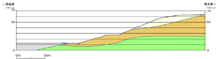
5号炉東側保管場所及び5号炉東側第二保管場所 斜面直交断面 (⑤断面)
