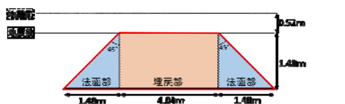
A-A' 断面
