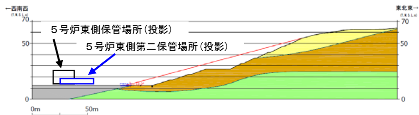
図 7-6 5号炉東側保管場所及び5号炉東側第二保管場所の周辺斜面崩壊後の土砂形状
