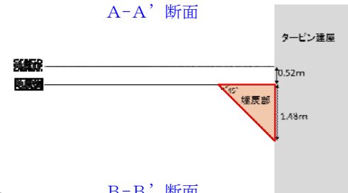
B-B' 断面
