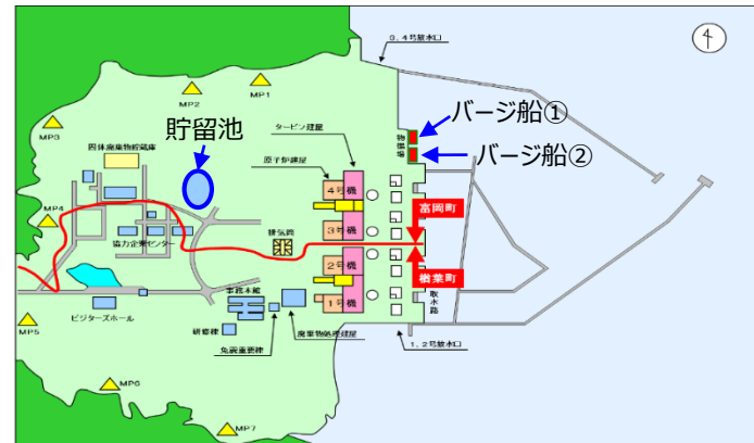
福島第二原子力発電所 現場概略図
